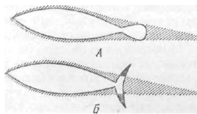
Рис. 67. Схема положения хвостового плавника различной формы относительно зоны вихрей и слоя трения (по Алееву):
