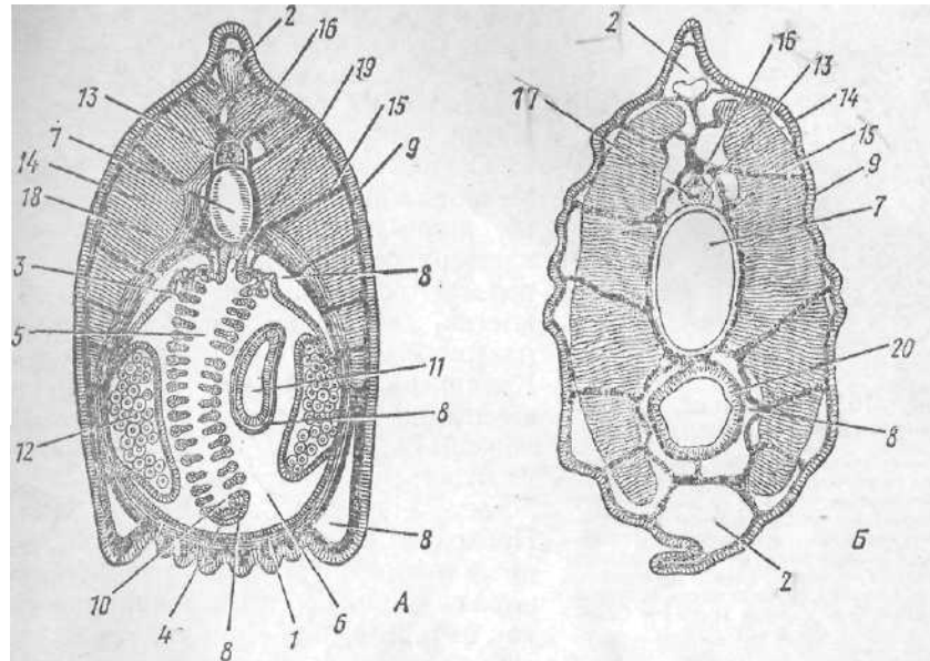
Рис 13. Поперечный разрез в жаберной области (А) и позади атриопора (Б):
