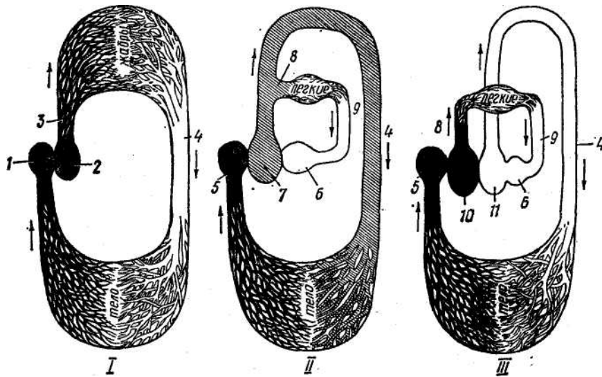
Рис. 46. Схема кровообращения позвоночных животных (по Бобринскому и Матвееву, 1966), / — первичноводное; // — земноводное; /// — высшее наземное позвоночное; черным цветом показана венозная кровь, белым — артериальная, штриховкой — смешанная.
