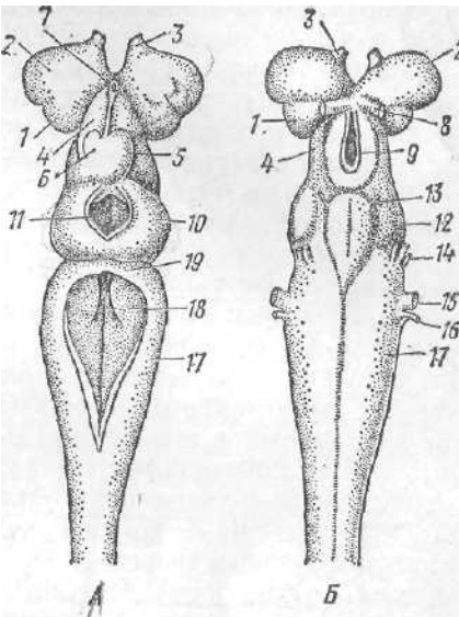
Рис. 63. Мозг миноги (по Паркеру), А — сверху; В — снизу:
