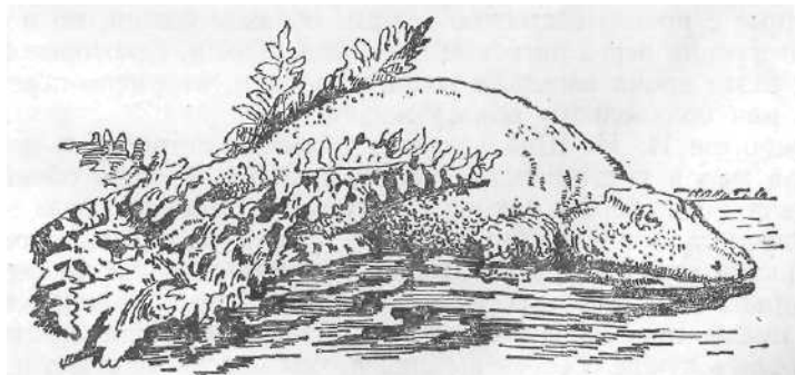
Рис. 145. Пермский рахитомовый лабиринтодонт — Eryops (по Шмальгаузену)
