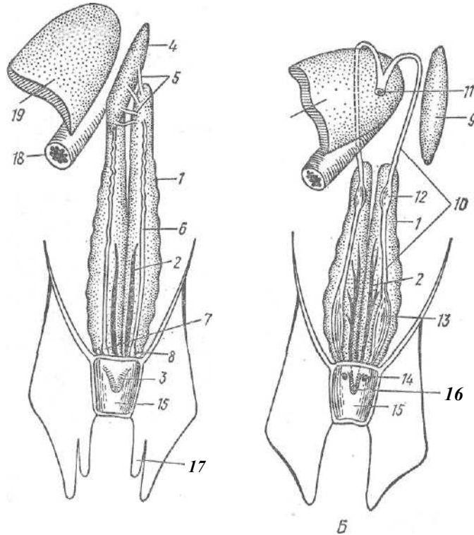
Рис. 89. Схема мочеполовой системы хрящевых рыб. А — самец; Б — самка:
