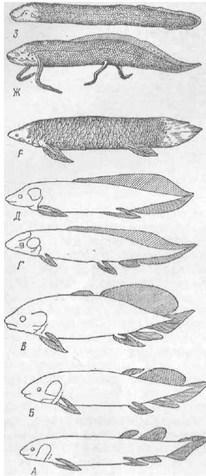
Рис. 76. Ископаемые и ныне живущие двоякодышащие рыбы.
