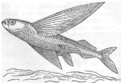
Рис. 104. Взлетающая четырёхкрылая летучая рыба — Cheilopogon pinnatibarbalus , справа схема взлета, вид сверху (по Шулейкину)
