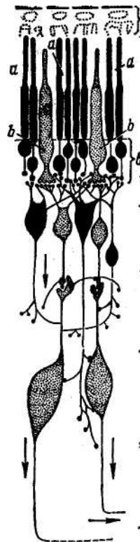
Рис. 37. Схематический разрез через сетчатку глаза (по Поляку):
