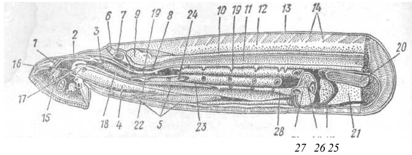
Рис. 54. Сагиттальный разрез головной части миноги:
