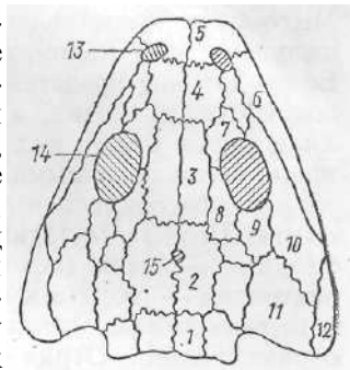
Рис. 144. Череп стегоцефала (по Шмальгаузену):
