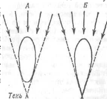
Рис. 109. Схема образования демаскирующей тени на брюхе рыбы (А). При брюшном киле (Б) тень на брюхе не образуется (по Алееву)
