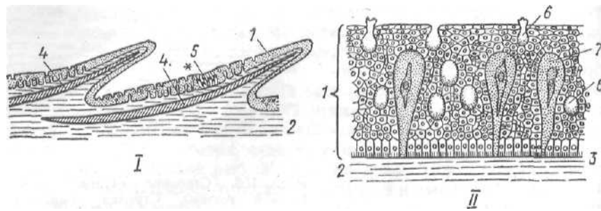
Рис. 107, Кожа костистой рыбы (по Гудричу). / — продольный разрез через участок с двумя чешуями; // — место, отмеченное на левом рисунке звездочкой (сильно увеличено):
