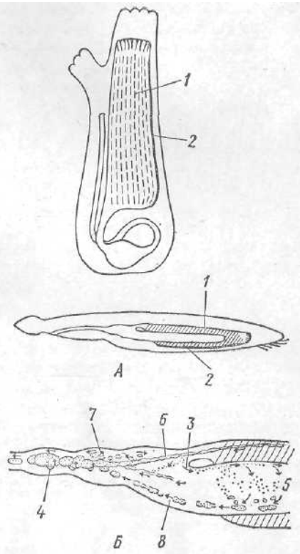
Рис. 16. Пищеварительная система ланцетника. А — Сходство с асцидиями (по Баррингтону, 1964); Б — средняя часть пищеварительной трубки и сложное движение в ней пищеварительных частиц (стрелки):
