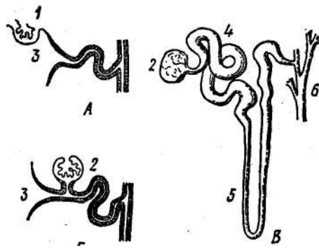
Рис. 47. Схемы почечных канальцев. А — предпочки с наружным клубком (1); Б — предпочки или первичной (туловищной) почки с внутренним клубком (2); В — тазовой почки, млекопитающего:
