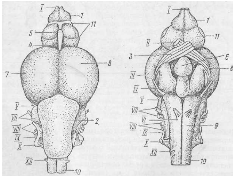
Рис. 129, Головной мозг форели сверху и снизу (по Видерсгейму);
