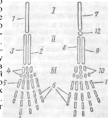
Рис. 152. Схема строения парных конечностей наземных позвоночных. А — передняя конечность; Б — задняя конечность:
