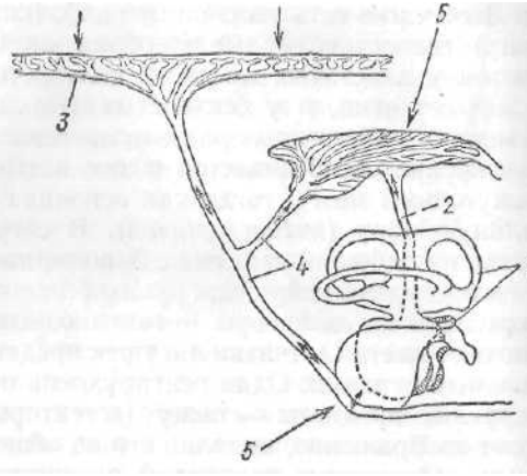
Рис. 170. Схема звукопередачи с венозной системы головы на внутреннее ухо хвостатых земноводных (по Шмальгаузену, 1964; упрощено):
