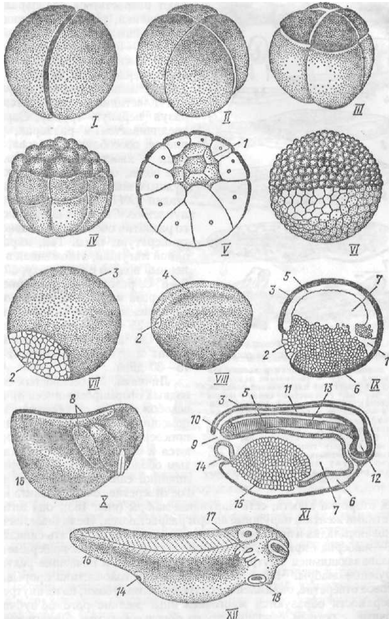
Ряс. 162. Развитие яйца лягушки (по Паркеру). Общий вид (стадии V, IX, XI — в разрезе); стадия XII — зародыш перед вылуплением: 1 — бластоцель, 2 — желточная пробка, 3 — эктодерма, 4 — медуллярная борозда, 5 — энтодерма, 6 — мезодерма, 7 — полость первичной кишки, 8 — впадины на месте будущих жаберных щелей, 9 — гастропор, 10 — нервно-кишечный канал, 11 — спинной мозг, 12 — головной мозг, 13 — хорда, 14 — район будущей клоаки, 15 — желточные клетки, 16 — хвост, 17 — наружные жабры, 18 — присоска
