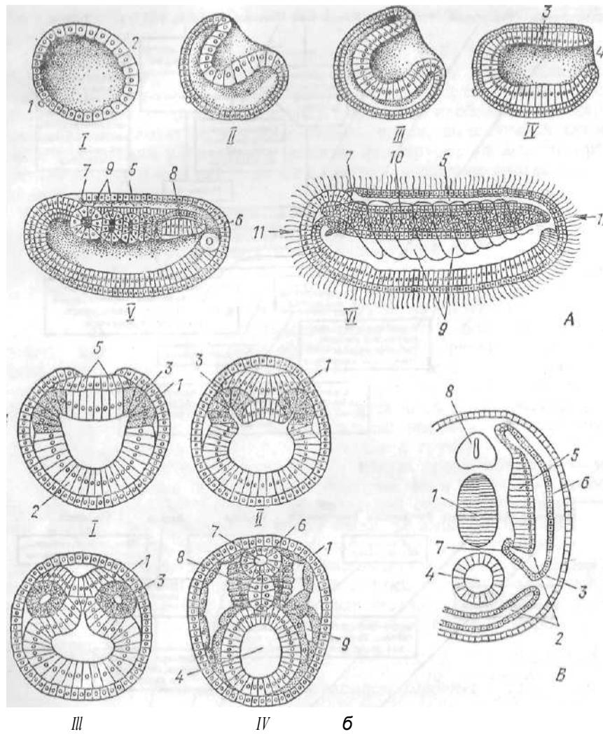
Рис. 6. Эмбриональное развитие хордовых животных (на примере ланцетника)
