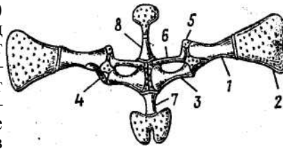
Рис. 153. Плечевой пояс лягушки (точками показан хрящ): 1 — лопатка, 2 — надлопаточный хрящ, 3 — коракоид, 4 — суставная впадина для головки плеча, 5 — прокоракоидный хрящ, 6 — ключица, 7 — грудина, 8 — предгрудинник
