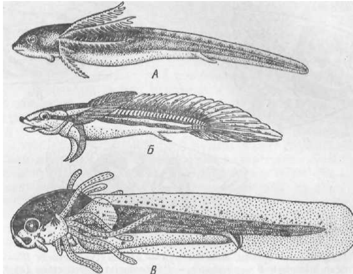
Рис. 117. Личиночные наружные жабры рыб (масштаб не соблюден; по Никольскому). А — американский чешуйчатник — Lepidosiren paradoxa ; Б — многопер — Polypterus sp.; В — вьюн — Misgurnus fossilis .
