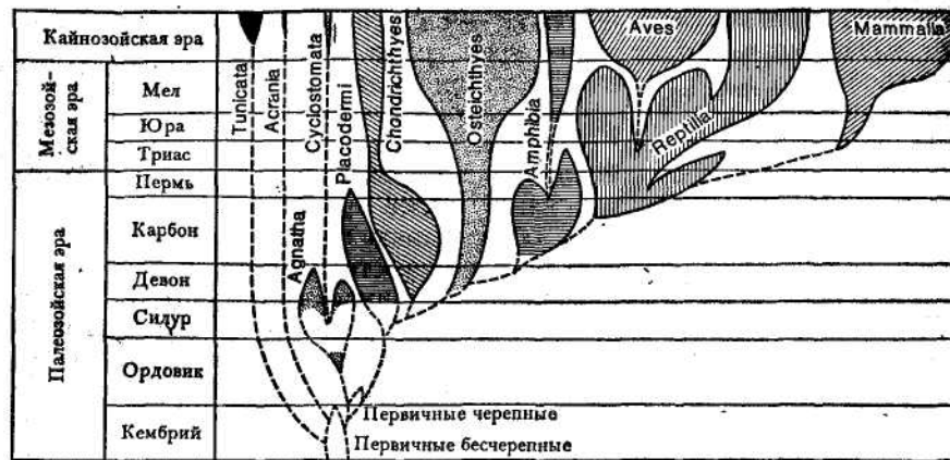
Рис. 49. Родословное дерево хордовых животных (по Матвееву, 1968, упрощено)
