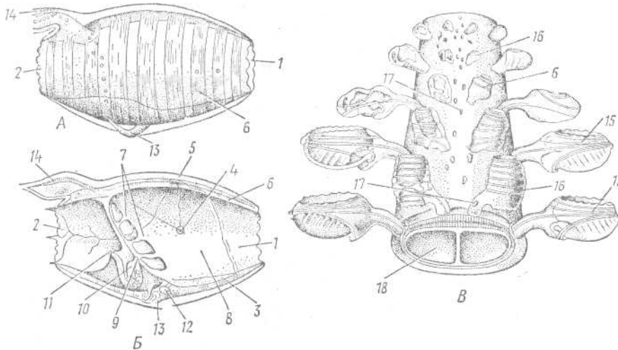
Рис. 28. Боченочник Dotiolum . А — внешний вид; Б — продольный разрез; В — спинной стolon с разными типами почек:
