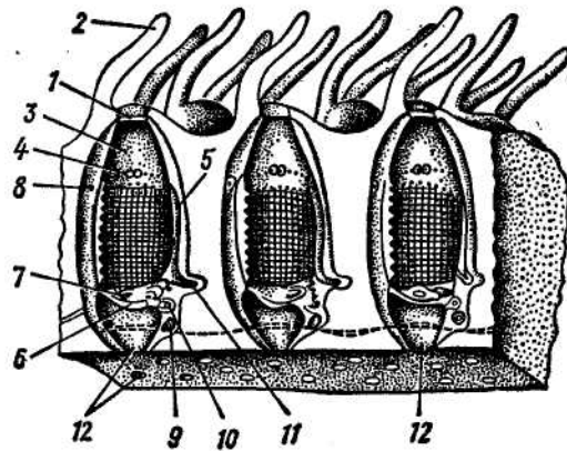
Рис. 26. Огнетелки Pyrosoma (часть колонии, видны зооиды):
