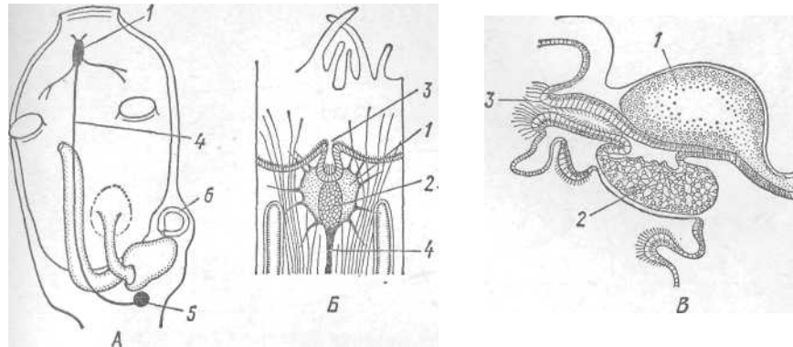
Рис. 22. Аппарат, синхронизирующий размножение одиночных асцидий Corella (по Хусу). А — схема связи гонад с нервным ганглием; Б, В — строение ганглионарного аппарата:
