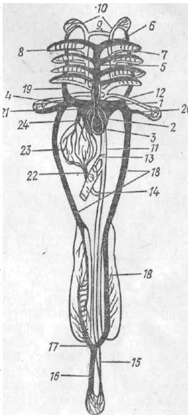
Рис. 120. Схема кровеносной системы костистой рыбы (черным цветом показаны сосуды с венозной кровью, белым — с артериальной):
