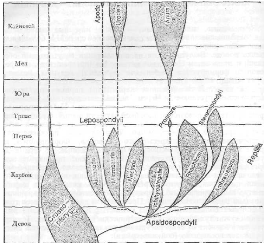
Рис. 143. Филогенетическое древо земноводных (по Ремеру и Шмальгаузену, с изменен.)
