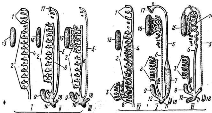
Рис. 48. Схема взаимоотношений половой и выделительной систем позвоночных животных (по Шмальгаузену, с изменен.) / — нейтральное зародышевое состояние; // — самка анамний; /// — самец анамний; IV — зародыш амниот; V — самка амниот; VI — самец амниот (пунктиром обозначены редуцирующиеся отделы):
