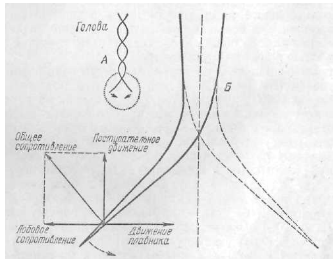
Рис 14. Перемещение ланцетника. А — движение тела; Б — движение хвостового отдела.
