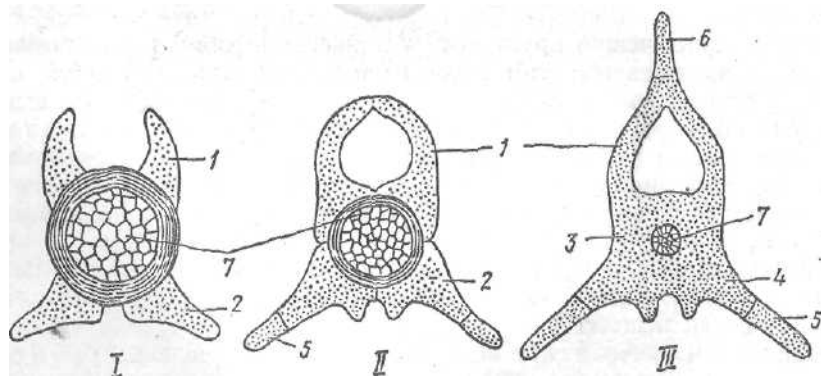
Рис. 81. Последовательные стадии развития (I—III) туловищного позвонка акулы (поперечные разрезы; по Щмальгауэену):
