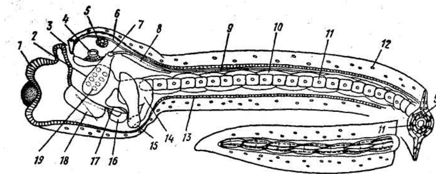
Рис. 23. Схема строения личинки асцидии Stavelina :
