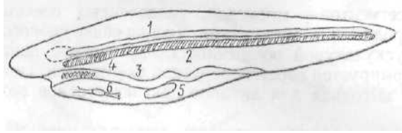
Рис. 7. Схема организации хордового животного:
