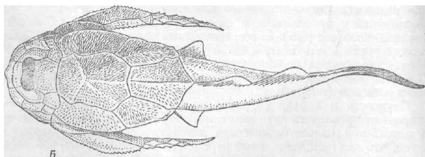
Рис. 70. Различные панцирные рыбы:
