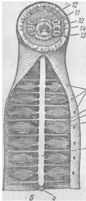
"3 Рис. 56. Положение жаберных мешков у миксины (А) и миноги (Б):
