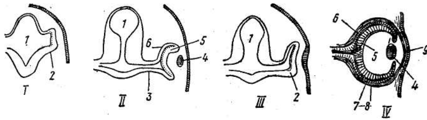
Рис. 38. Последовательные стадии развития глаза (I—IV — схема) (по Шмальгаузену):
