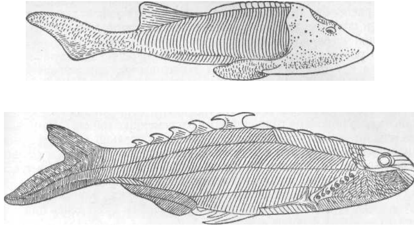
Рис. 52. Cephalaspis (Osteostraci) (4). Нижний девон; Birkenia (Anaspida) (5), силур, реконструкция
