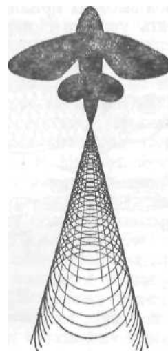
Рис. 104. Взлетающая четырёхкрылая летучая рыба — Cheilopogon pinnatibarbalus , справа схема взлета, вид сверху (по Шулейкину)
