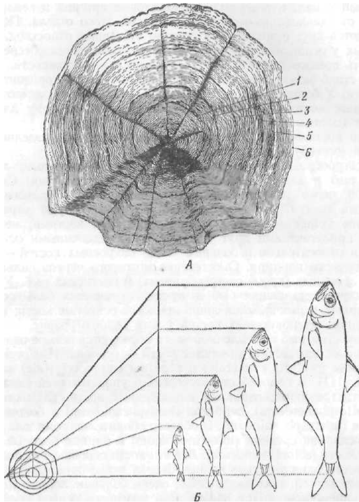
Рис. 110. Чешуя воблы с годовичными кольцами (А) и соотношение изменения размеров чешуи и длины рыбы (Б) (по Никольскому): 1—6 — годовые слои
