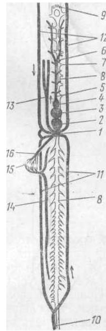
Рис. 59. Схема кровеносной системы невольской миноги (вид с брюшной стороны; по Гуртовому):
