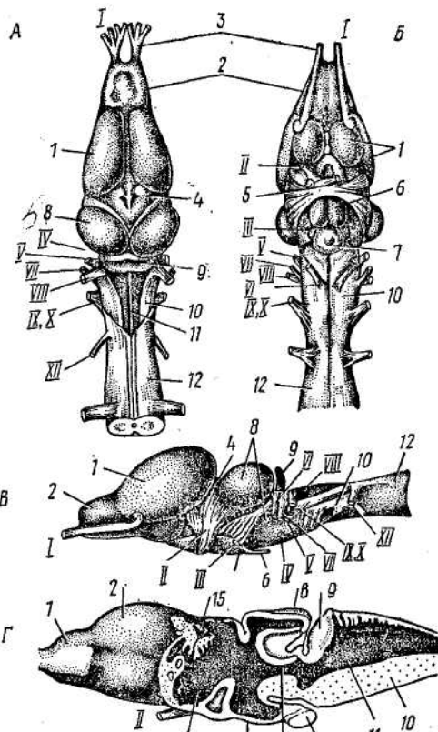
Рис. 168. Головной мозг лягушки (по Паркеру). А — сверху; Б — снизу; В — сбоку; Г — в продольном разрезе:
