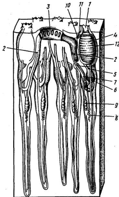
Рис. 25. Колониальная (сложная) асцидия (участок колонии):
