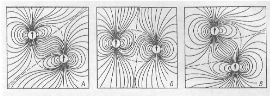
Рис. 138. Силовое поле вокруг двигающихся рыб. А — рыбы взаимно притягиваются; Б — рыбы не влияют друг на друга; В — рыбы взаимно отталкиваются (по Шулейкину)
