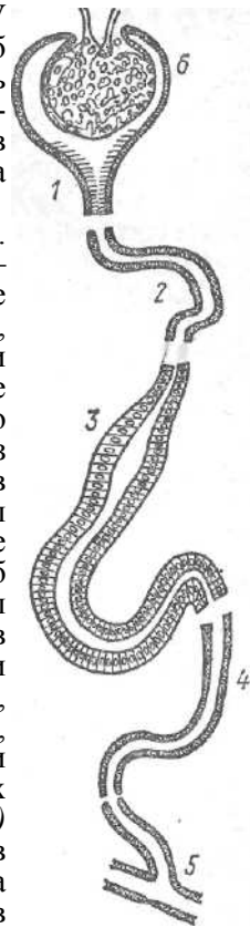
Рис. 90. Строение почечного канальца акулы (по Борсез):
